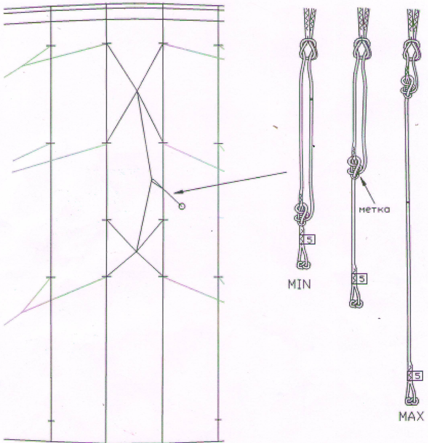
Юп II Регулировка длины пятой стропы
