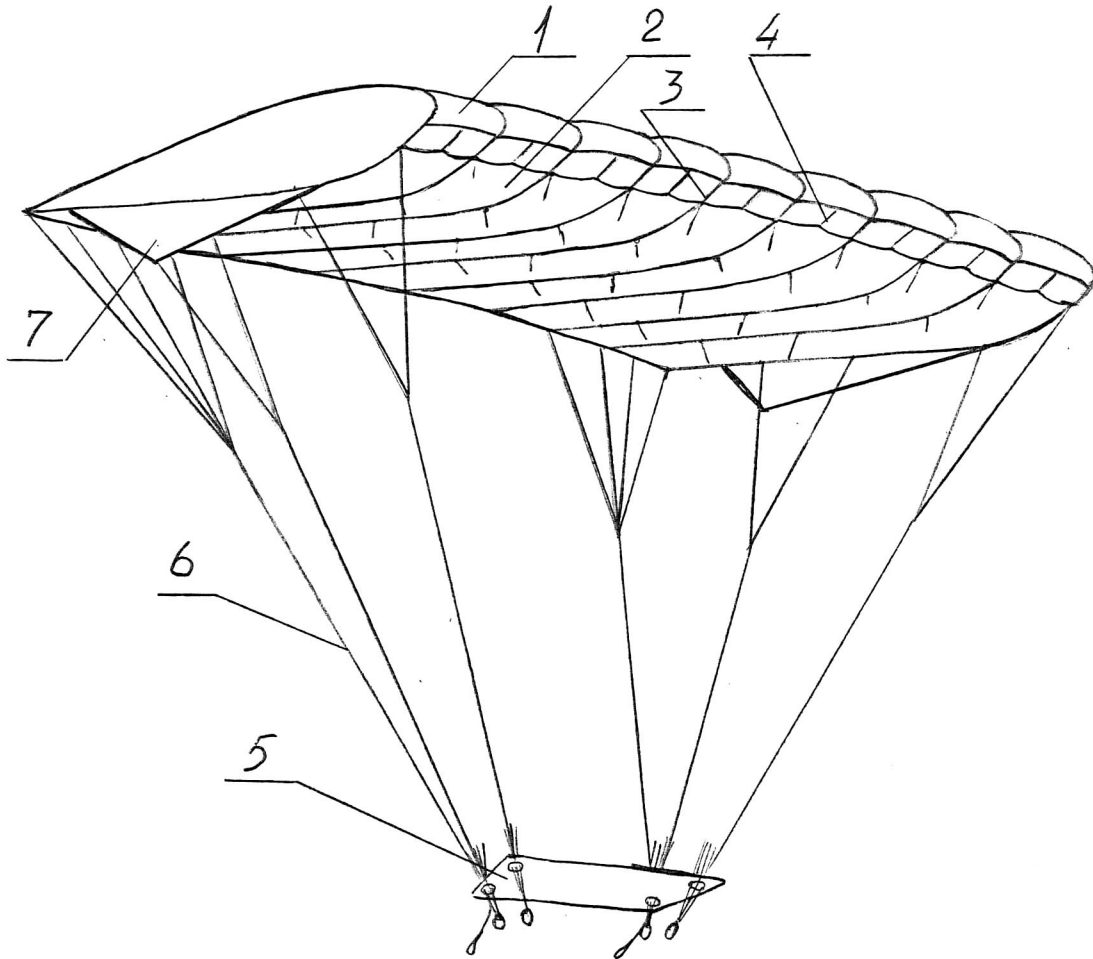
Рис. 1. Парашют «Ultimate»:
